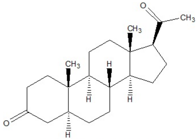
5alpha-Pregnane-3,20-dione
