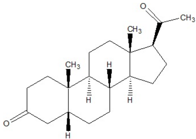
5beta-Pregnane-3,20-dione
